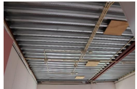
Onderkant van het gegalvaniseerde dak
